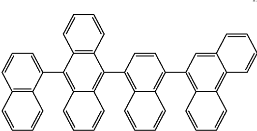
H16
