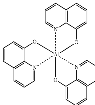
Alq 3
