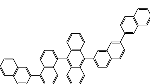
H16
